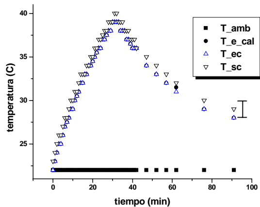
Fig.2.- Ciclo típico de calentamiento-enfriamiento.
