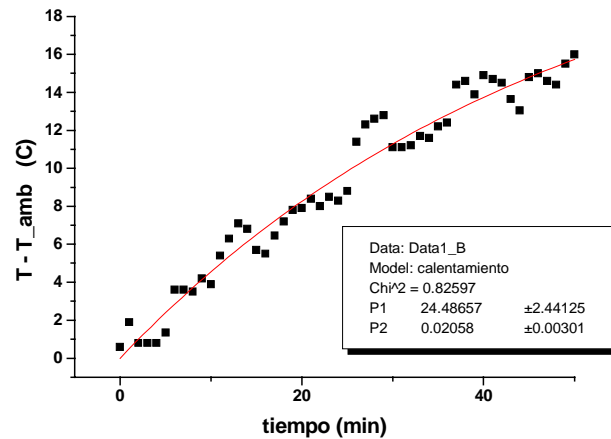
Fig.4.- Ajuste de datos experimentales con radiación solar como fuente de calor.
