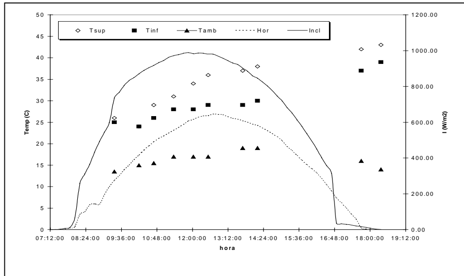
Fig.2.- Evolución de las temperaturas del agua y ambiente y de Intensidad de radiación solar incidente.
