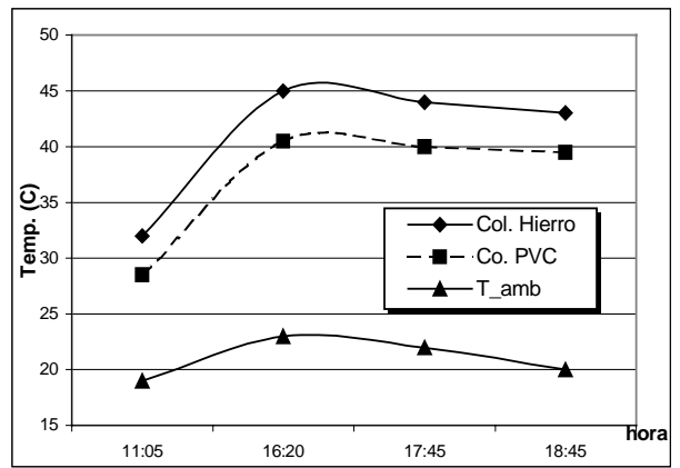
Fig.4.- Evolución de temperatura para tubo colector de distinto material, PVC y hierro galvanizado.
