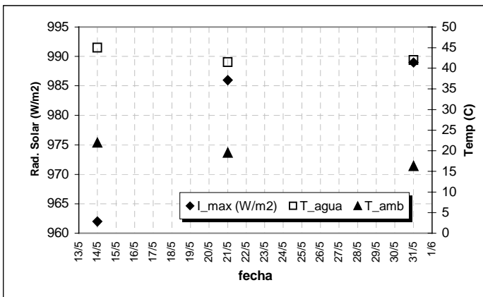
Fig.3.- Valores máximos de Intensidad de radiación solar y temperaturas medias registradas.
